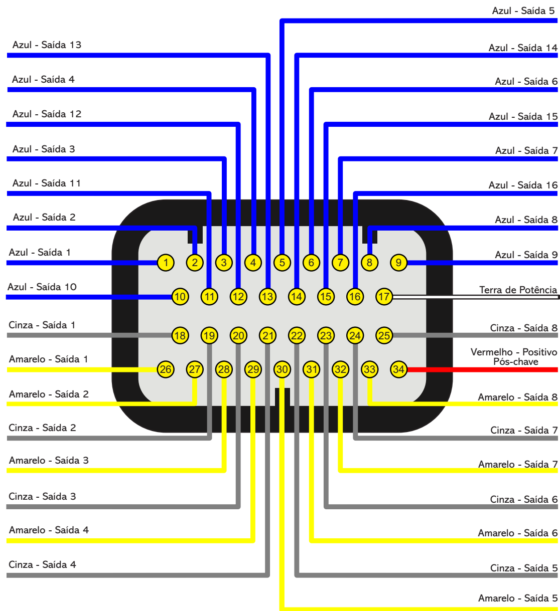
Vista traseira do conector
